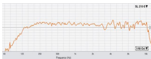
Resposta de frequência
